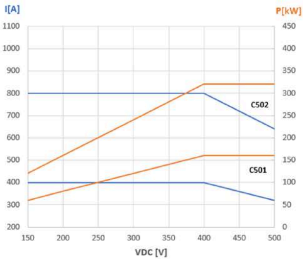
Figura 2. Curva di potenza (funzionamento continuo)
